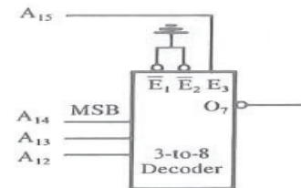
Using Decoder
